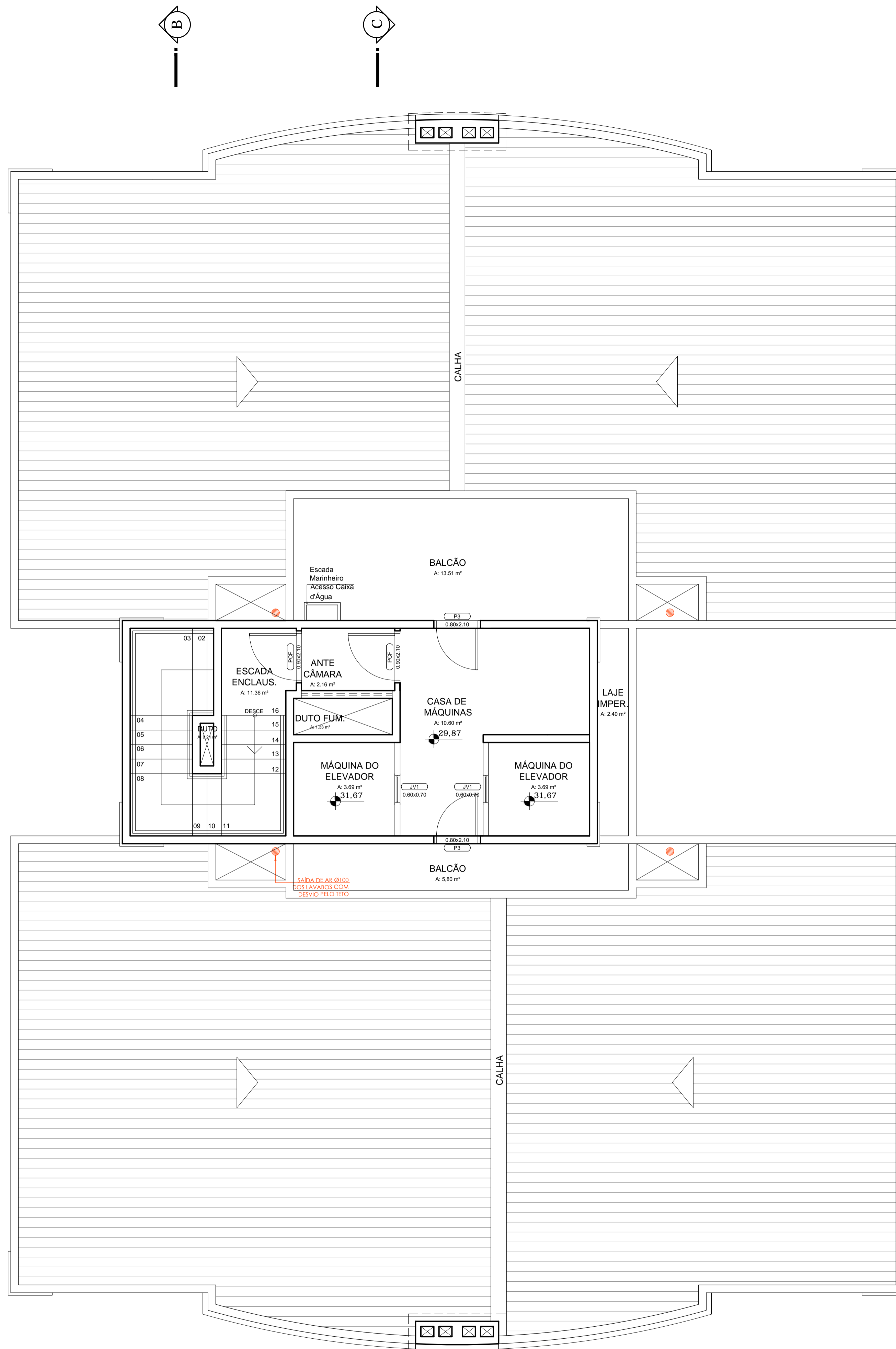
PLANTA BAIXA PAVTO CASA DE MÁQUINAS - TORRE 03/ 04/ 05/ 06/11/ 12 ÁREA DO PAVTO: 48,82m 2
